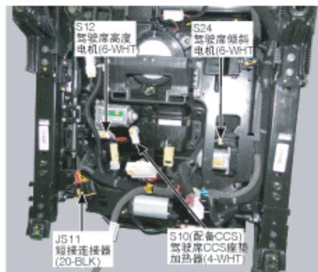
194. 驾驶席座椅
