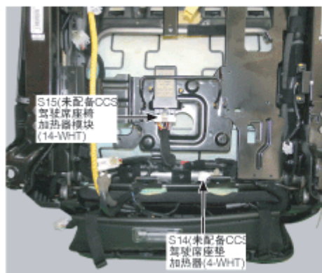
196. 驾驶席座椅
