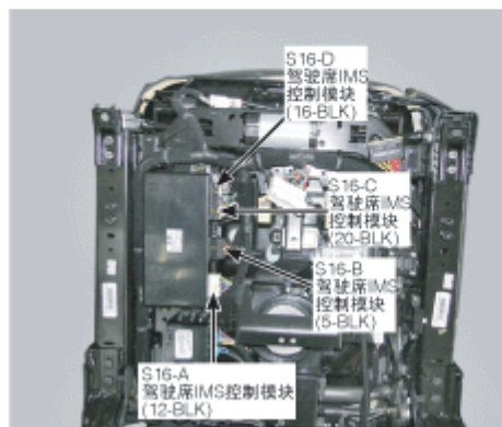
193. 驾驶席座椅
