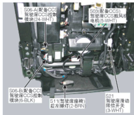
195. 驾驶席座椅
